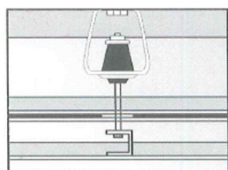
Plafonds acoustiques
